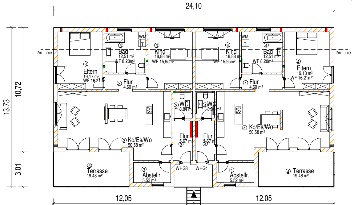
Grundriss OG
