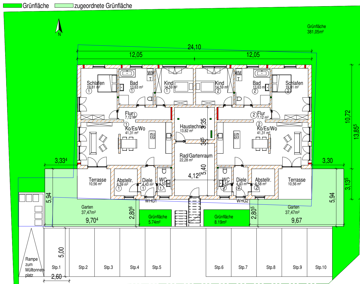
Grundriss EG
