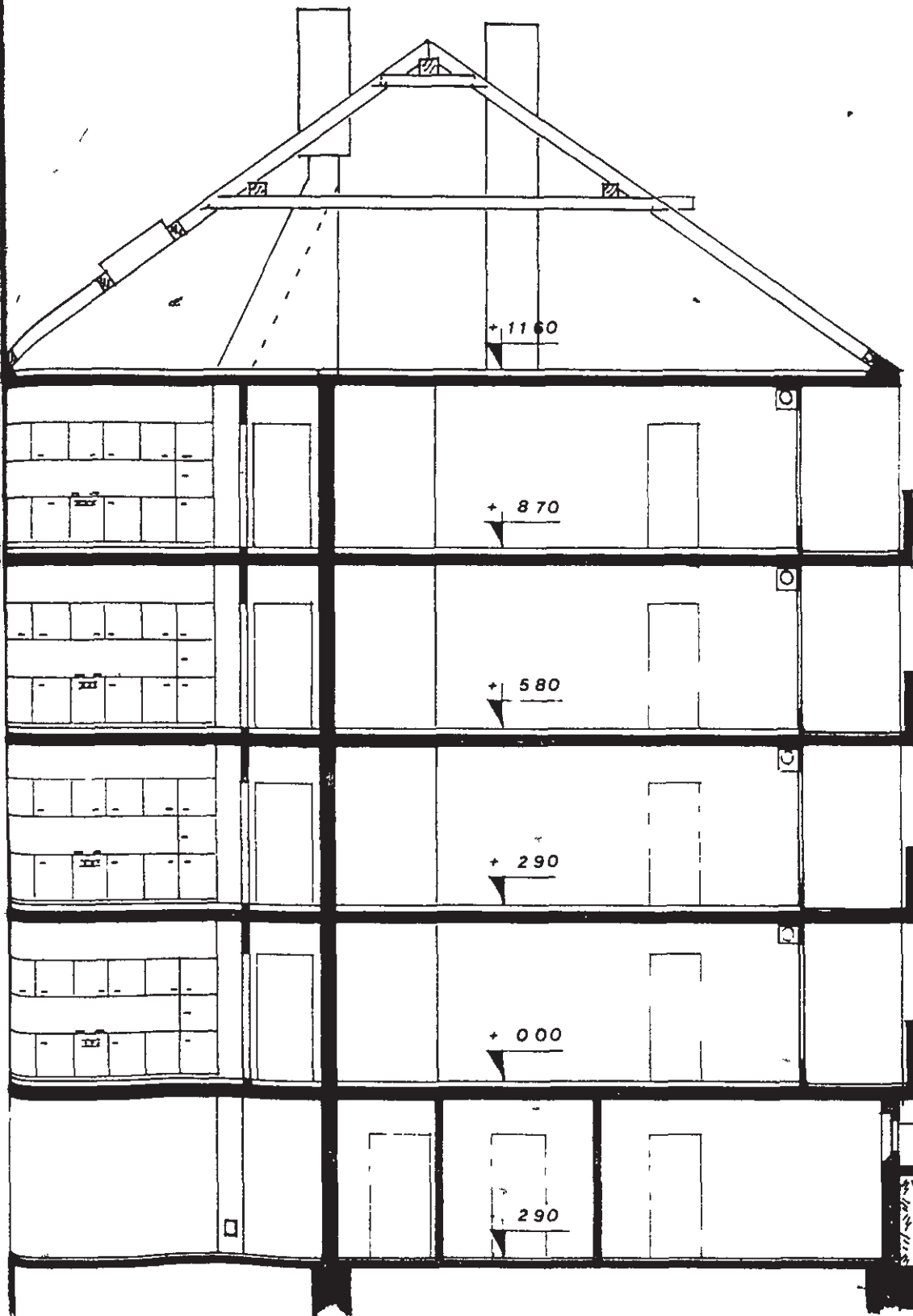
SCHNITT HAUS 3 C-D
