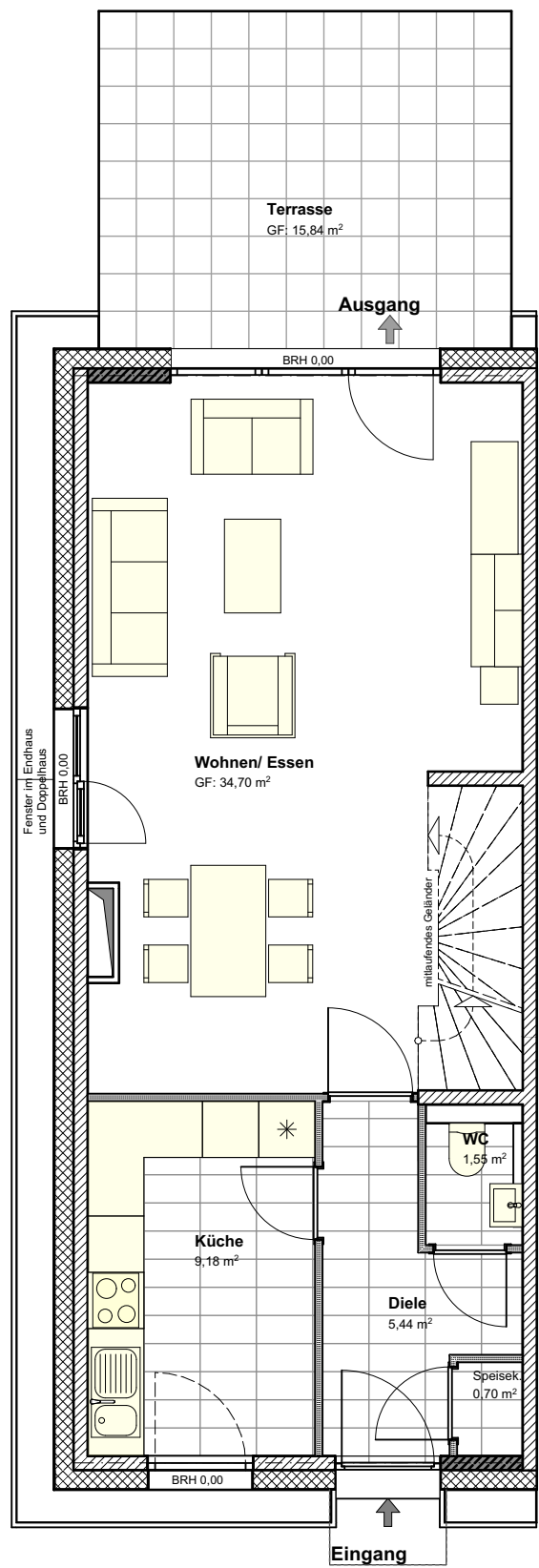
ERDGESCHOSS
