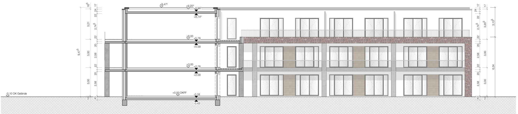
Schnitt B-B
