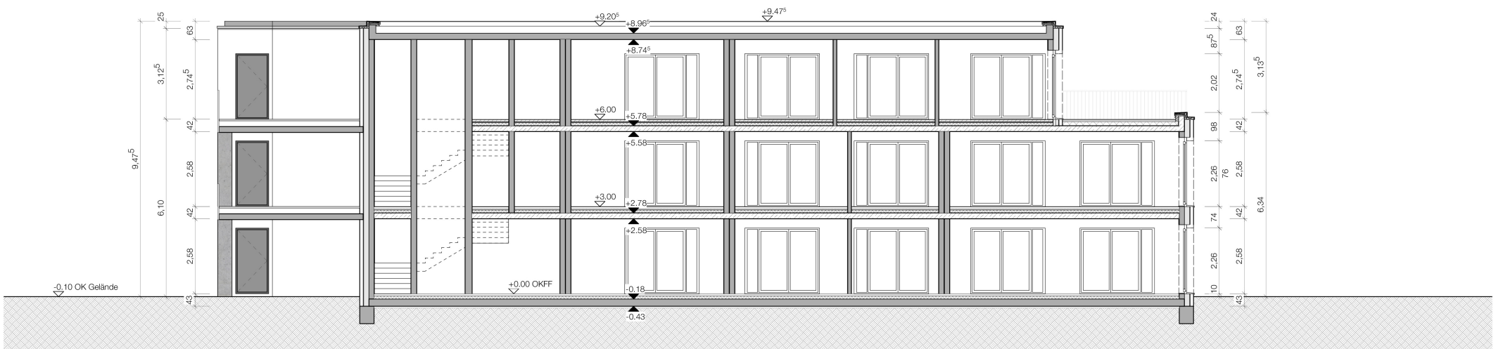
Schnitt A-A
